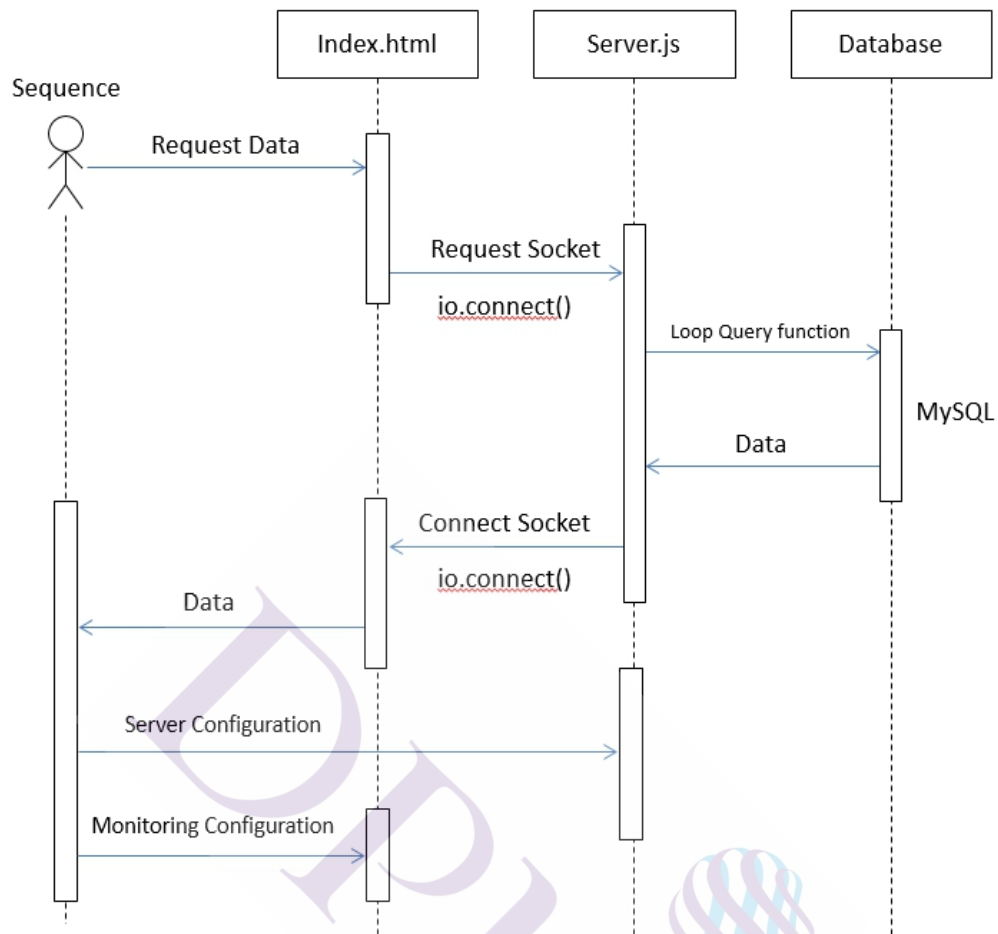
ภาพที่ 3.37 แผนภาพลำดับขั้นตอนของผู้ดูแลระบบในส่วนตรวจสอบความผิดปกติของระบบ
