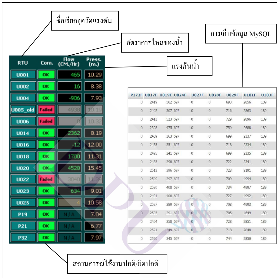
ภาพที่ 2.5 หน้าจอระบบสถานีที่ศูนย์ควบคุมหรือสถานีหลัก (Master Station) และฐานข้อมูล
