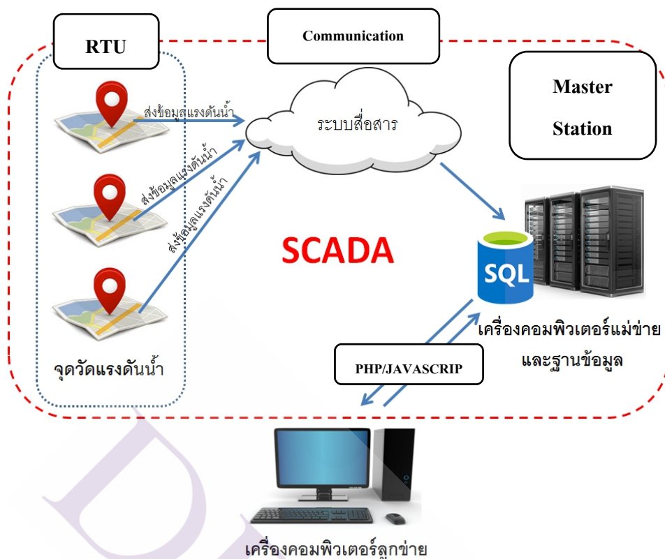
ภาพที่ 2.4 ภาพรวมของระบบสกาด้าเมื่อนำมาใช้กับโปรแกรมตรวจสอบแรงดันน้ำ
