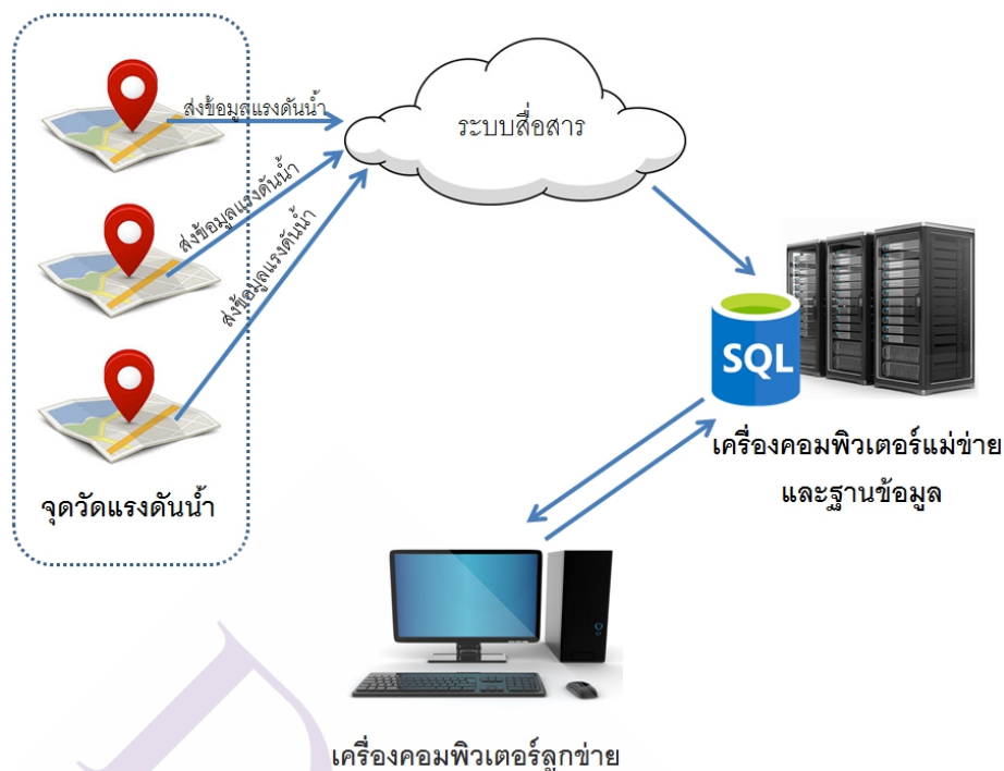
ภาพที่ 1.1 ภาพรวมของระบบการรับส่งข้อมูลแรงดันน้ำ
