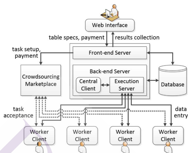
ภาพที่ 2.8 ภาพรวมโครงสร้างการทำงานของระบบโครวด์ฟิลล์ (Crowd Fill) 3
