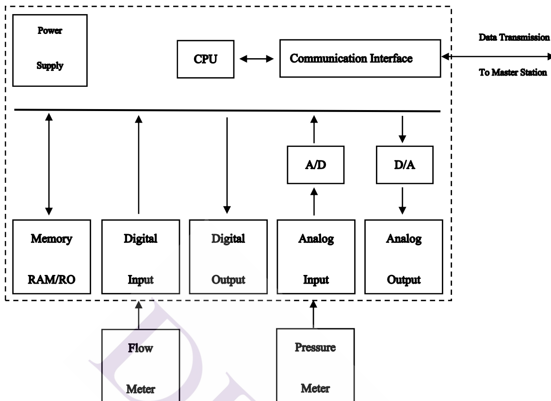
ภาพที่ 2.3 การเชื่อมต่อระหว่างหน่วยควบคุมระยะใกล้กับเครื่องมือวัดภาคสนาม
