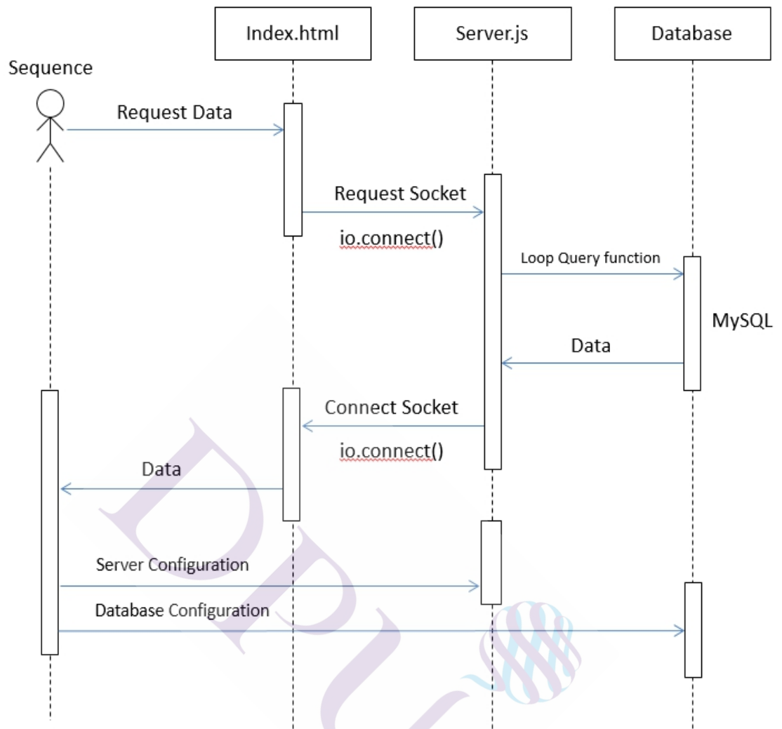
ภาพที่ 3.38 แผนภาพลำดับขั้นตอนของผู้ดูแลระบบในส่วนตั้งค่าใช้งานของระบบ
