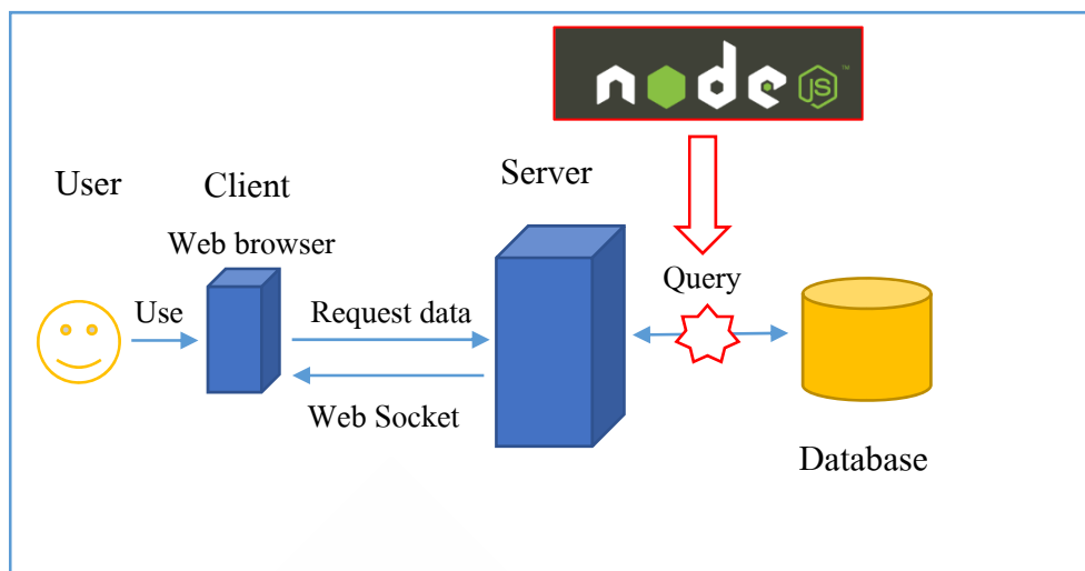
ภาพที่ 3.5 หลักการทำงานของการทำงานเขียนโปรแกรมภาษาโนดคือทเจเอส
