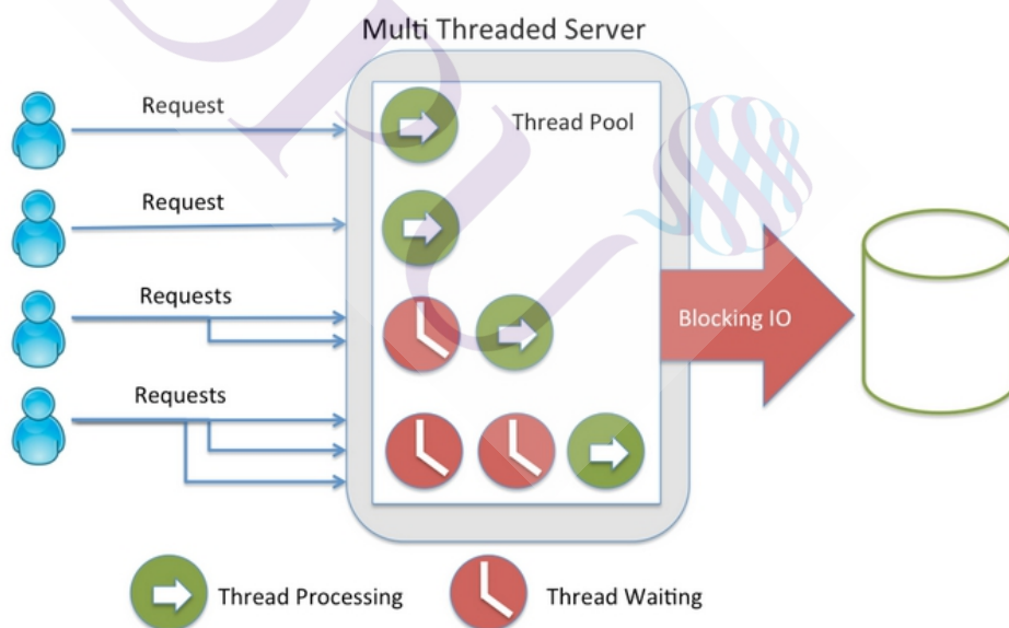
ภาพที่ 2.7 โครงสร้างการทำงานแบบแม่ข่ายมัลติเทร็ด (Multi-Threaded Server) 2
