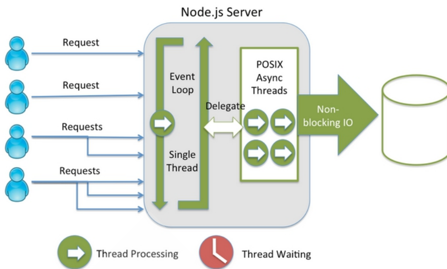
ภาพที่ 2.6 โครงสร้างการทำงานของแม่ข่ายโนดคือทเจเอส (Node.js Server) 2
