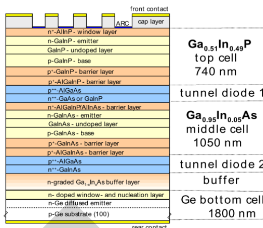
รูปที่ 2.27 เซลล์แสงอาทิตย์แบบ multifunction solar cells
