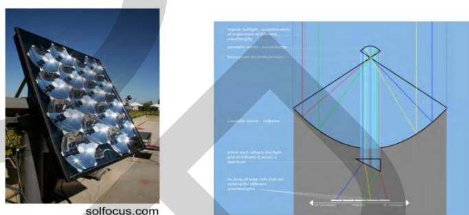
รูปที่ 2.23 CPV แบบ parabolic refractor
