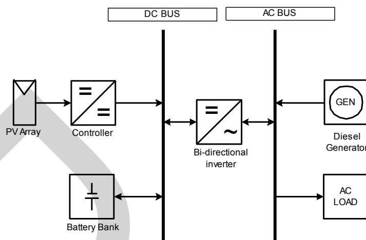
รูปที่ 2.12 ระบบผลิตไฟฟ้าแบบผสมผสานแบบขนาน
