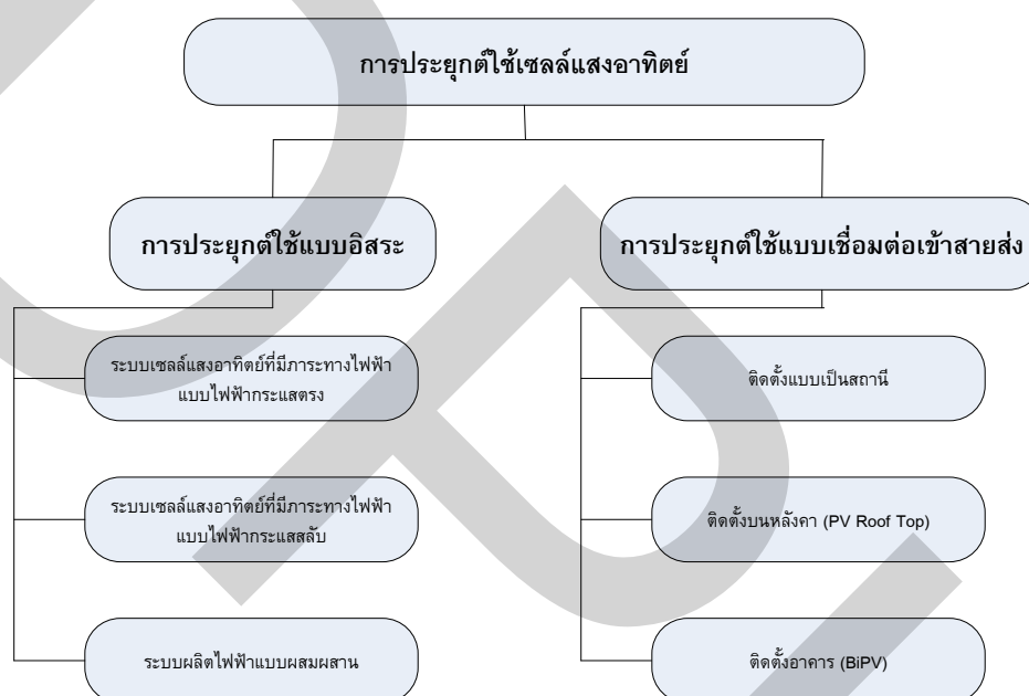
รูปที่ 2.3 การจำแนกการประยุกต์ใช้พลังงานแสงอาทิตย์ในรูปของไฟฟ้า
