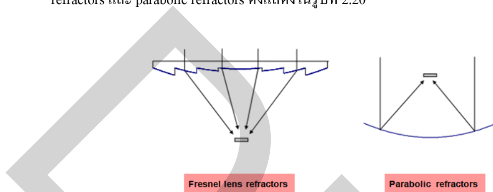
รูปที่ 2.20 การรวมแสงของ CPV
